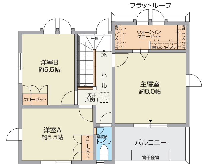
2F
